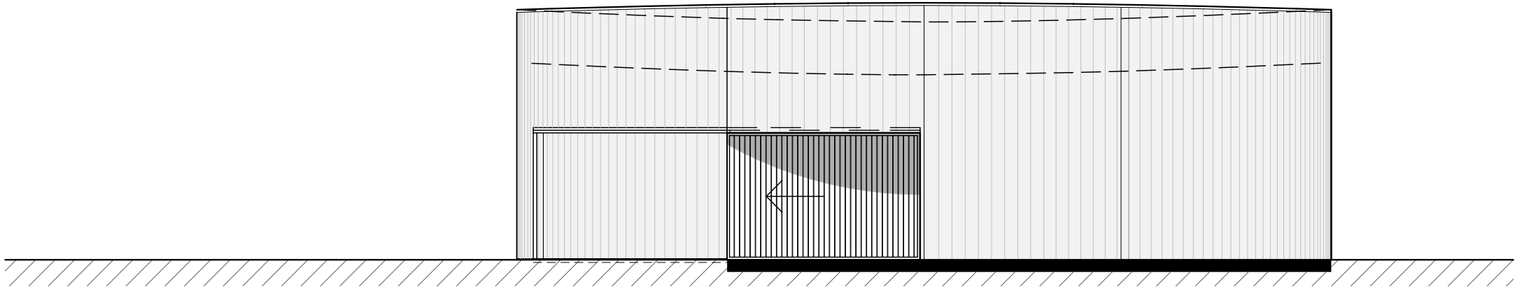
CRNG LOCAL VOILE ELEVATION SUD 1:100
