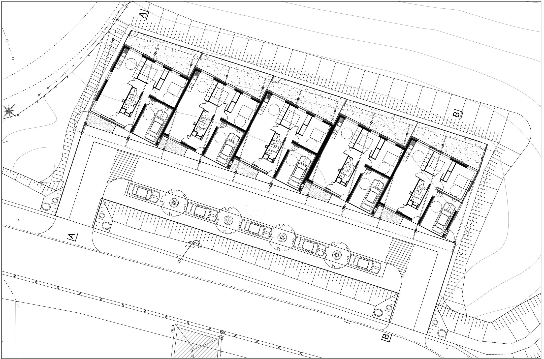
PLAN REZ-DE-CHAUSSEE
