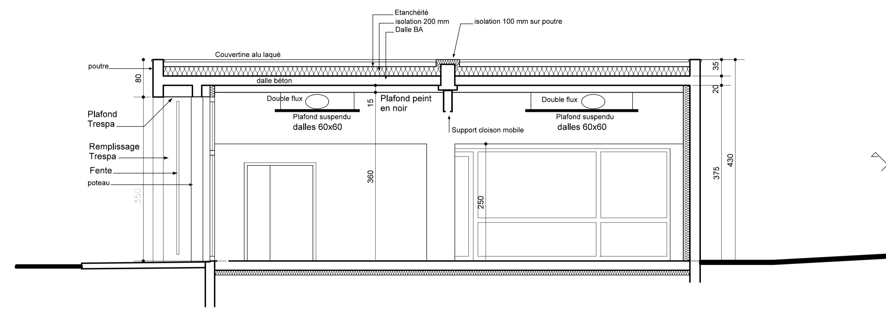
Coupe D-D
