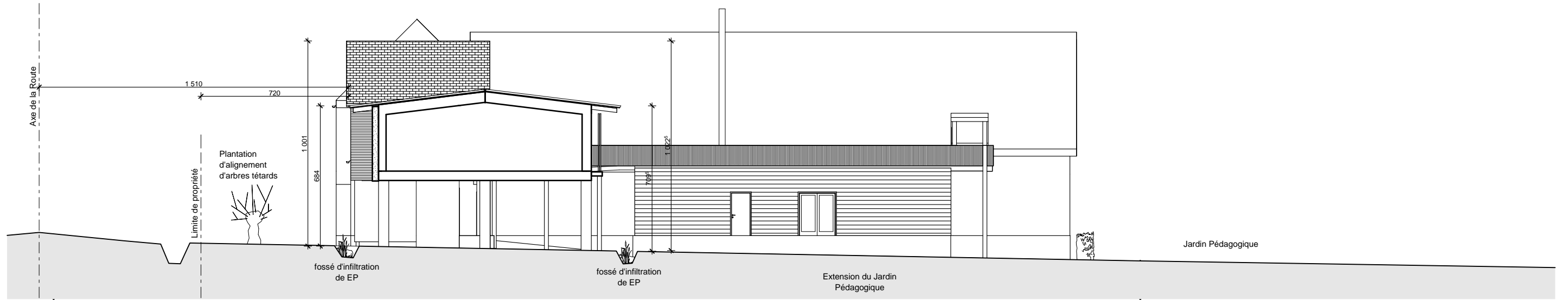
Coupe paysagère
