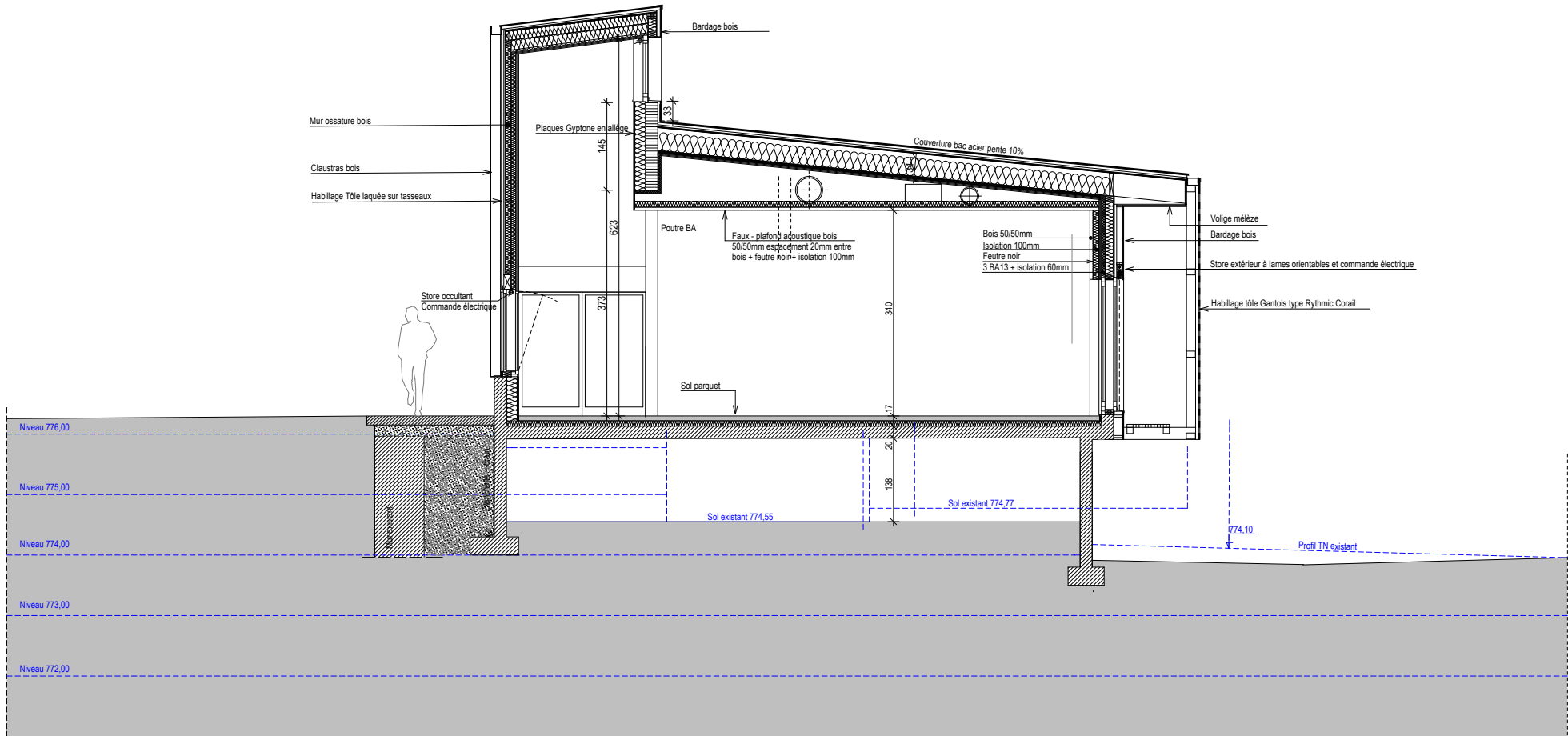
Coupe transversale
