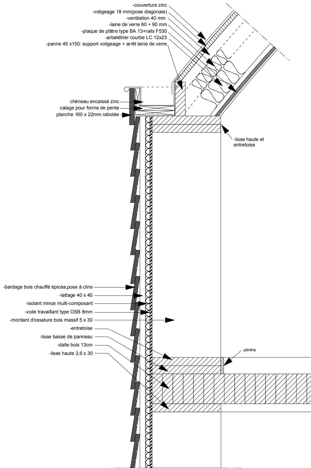
COUPE SUR MUR éch. 1/10
