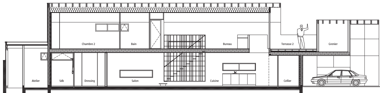
Coupe longitudinale.
