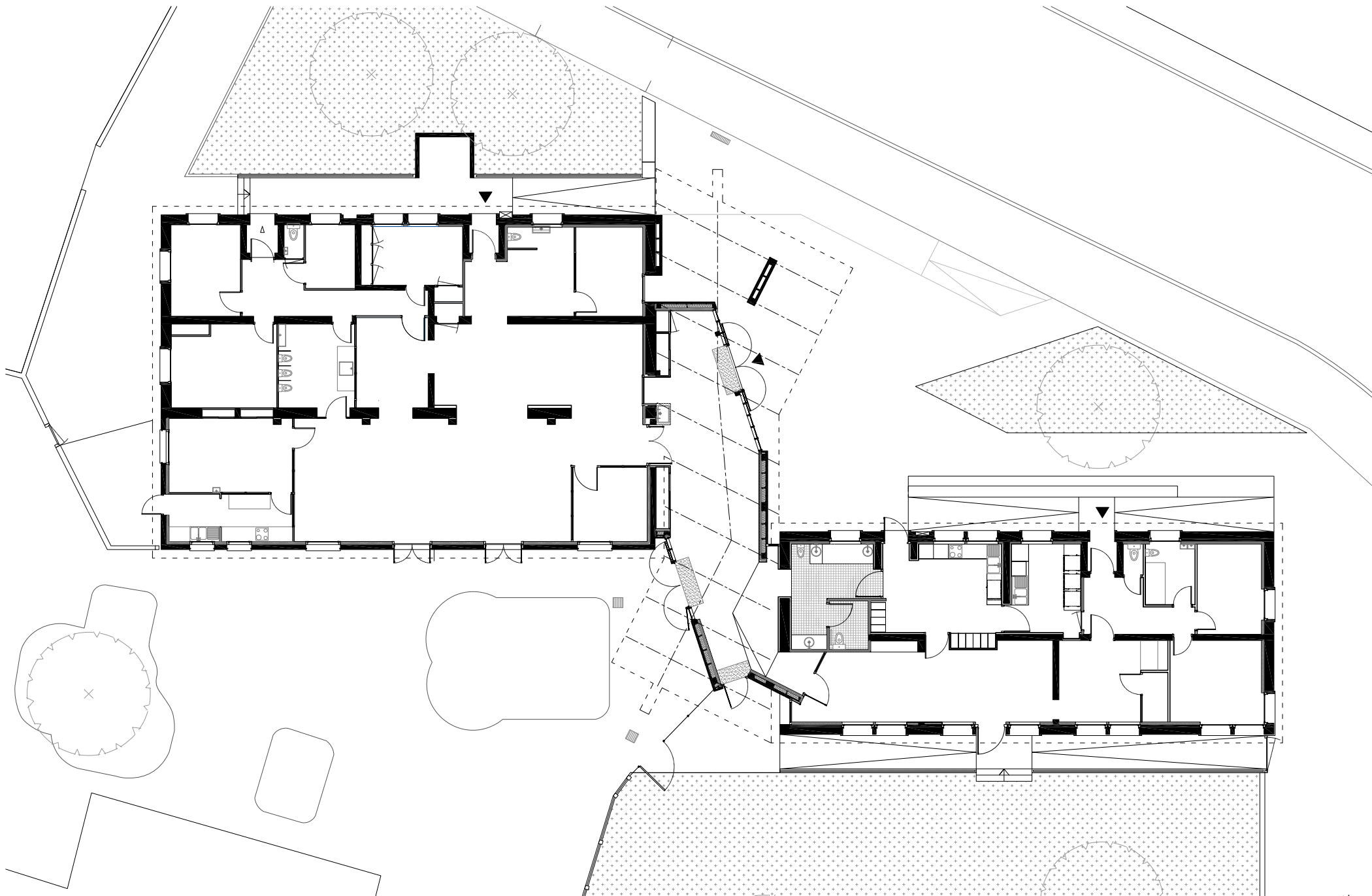
Multi-accueil 'Bout d'Chou' - Donges (44) - Plan RdC
