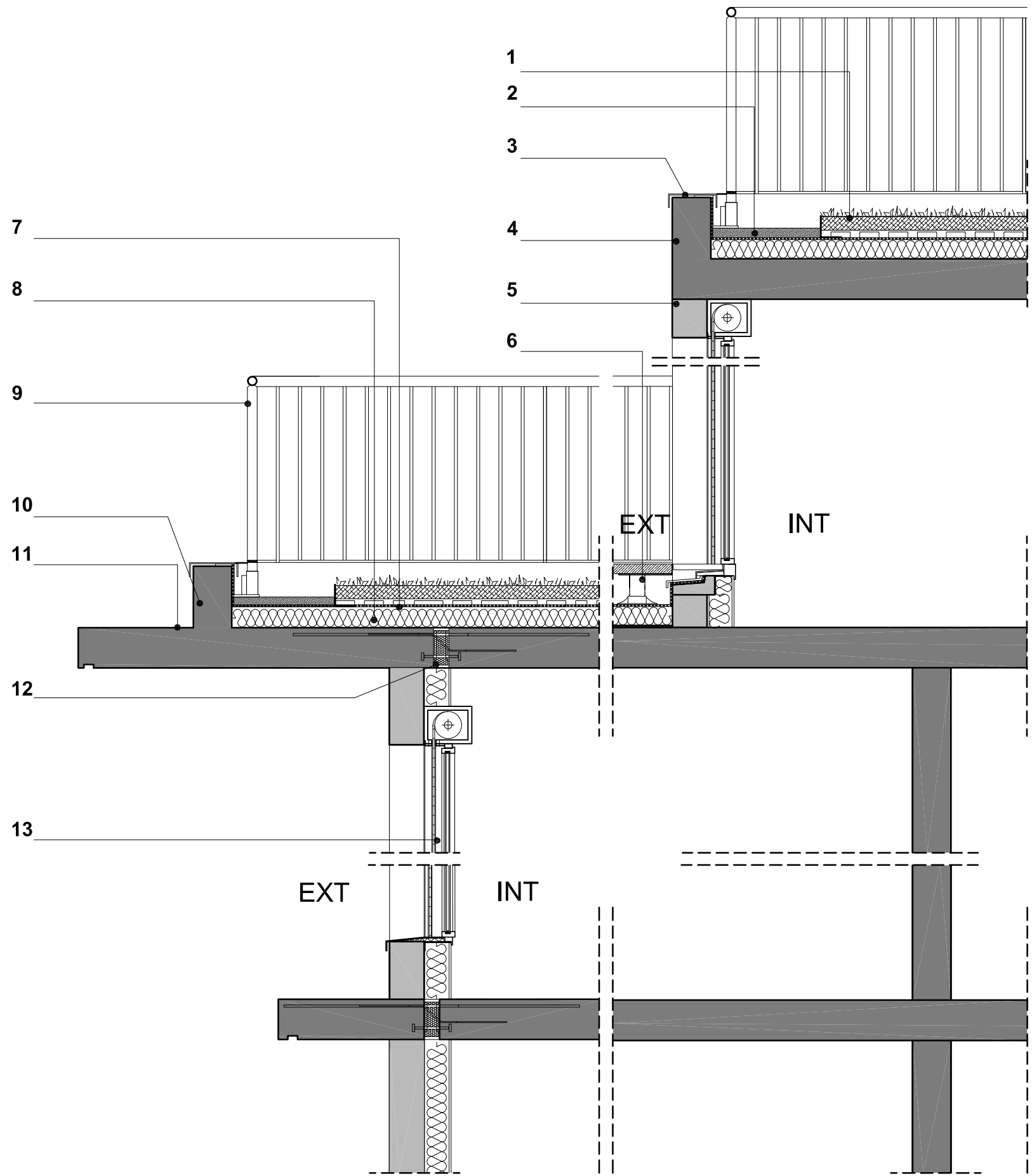
Détail sur terrasse
