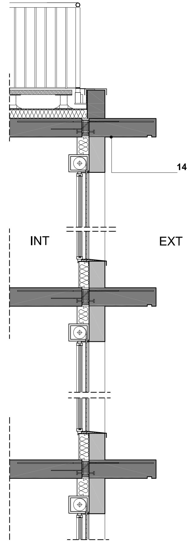
Détail façade type
