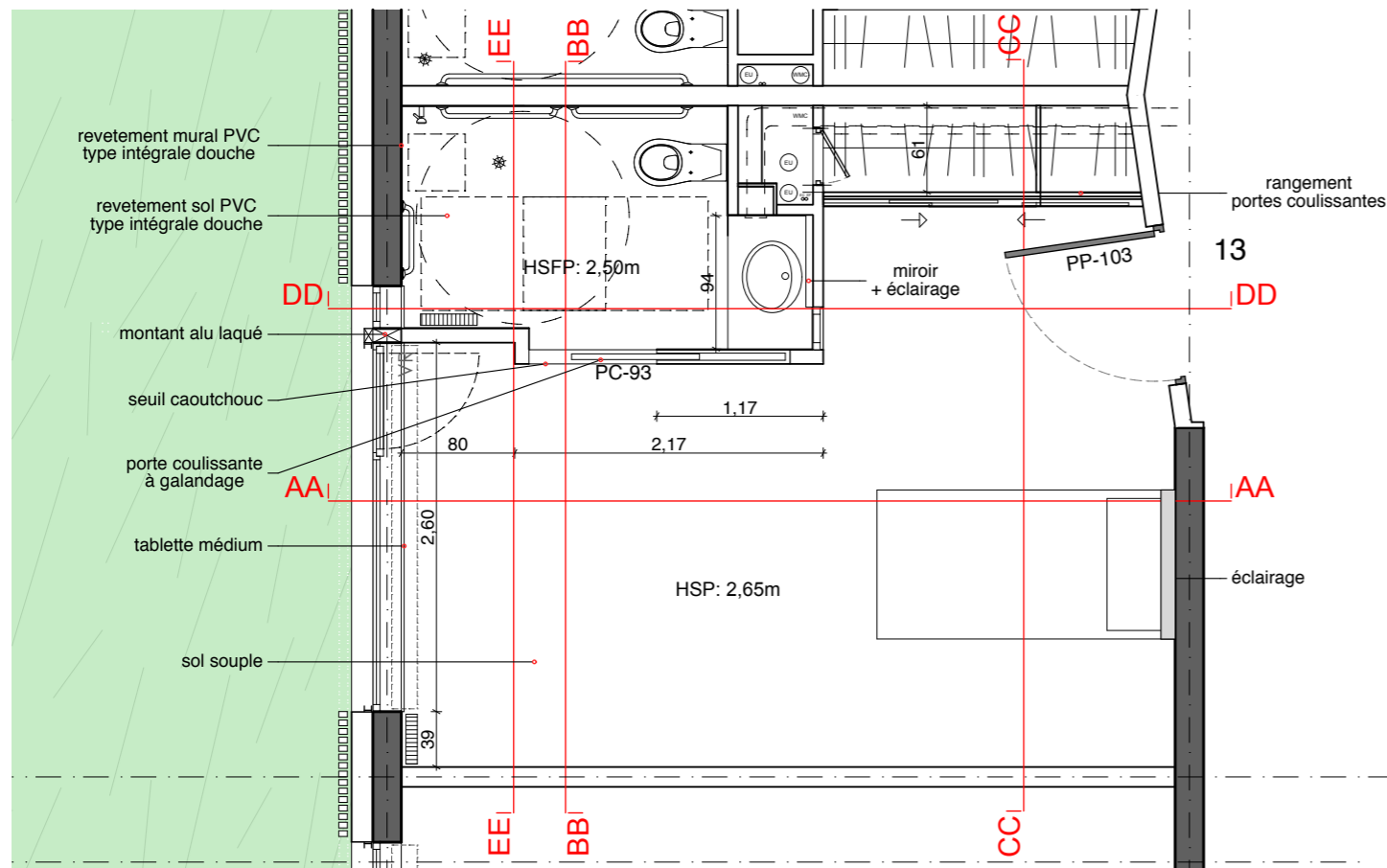
PLAN RDC
