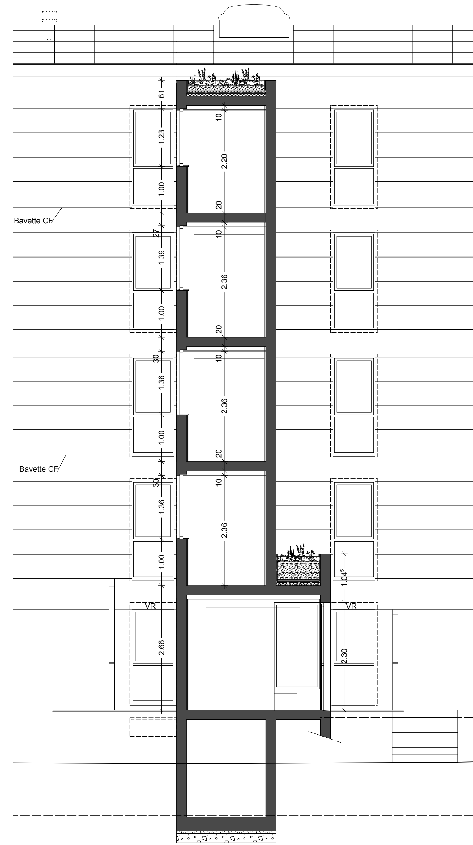
Coupe C-C
