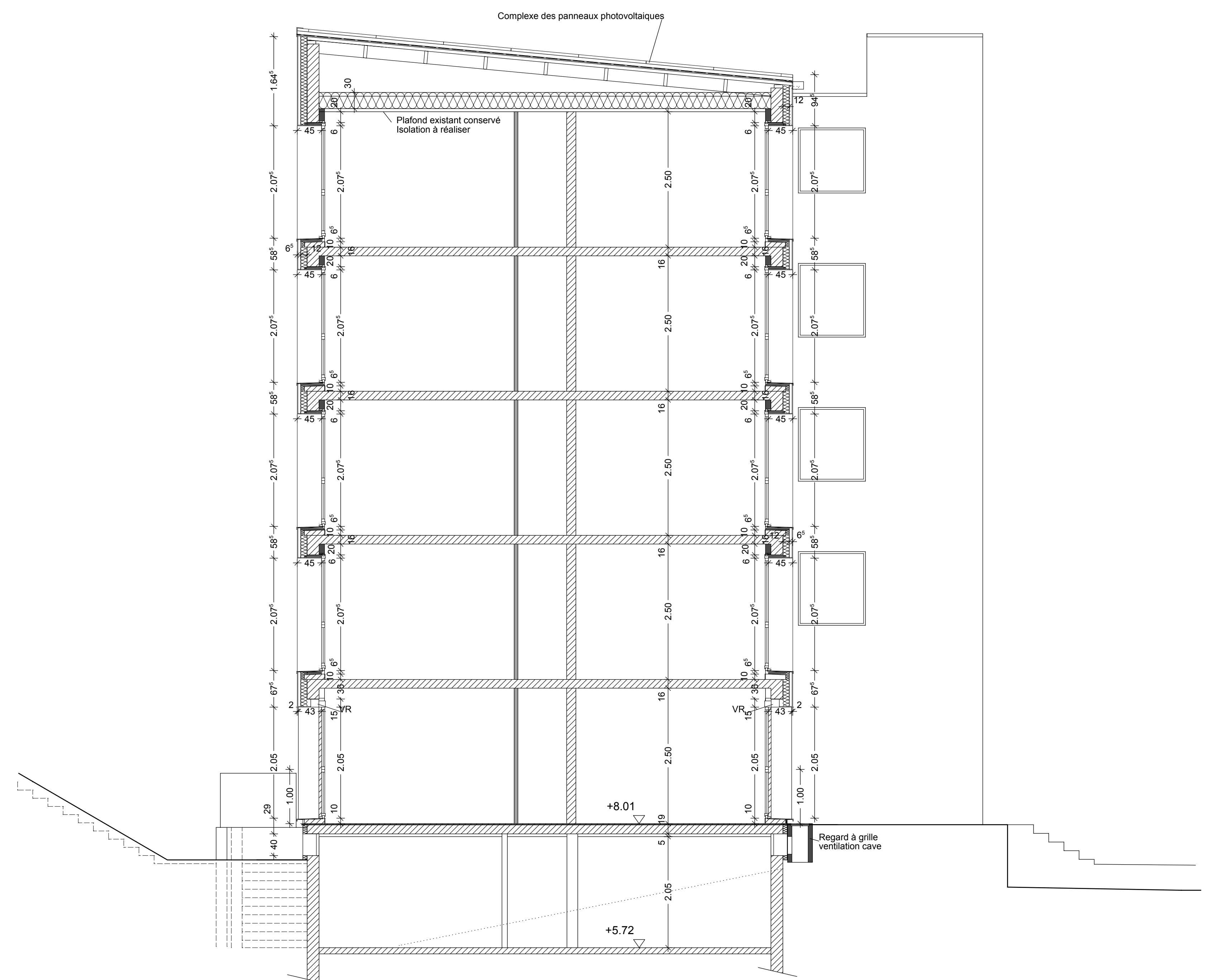
Coupe D-D
