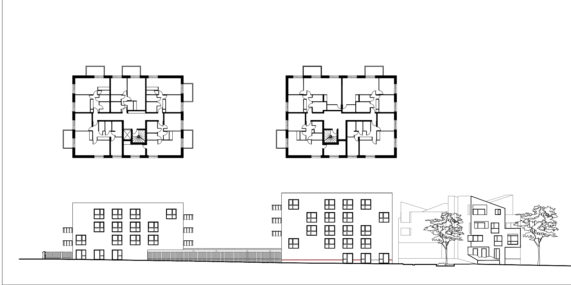
ELEVATION ET PLAN D'ETAGE COURANT
